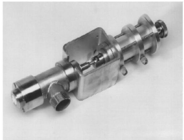
2 – Sitz - Dosierventil
