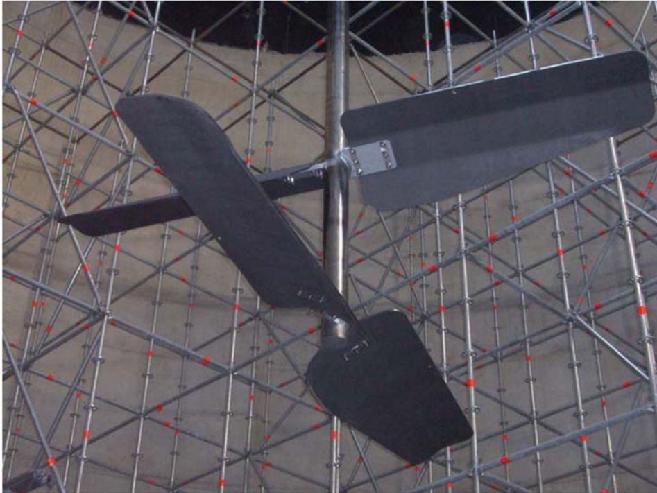
4 flügeliges Hydrofoil Rührelement
